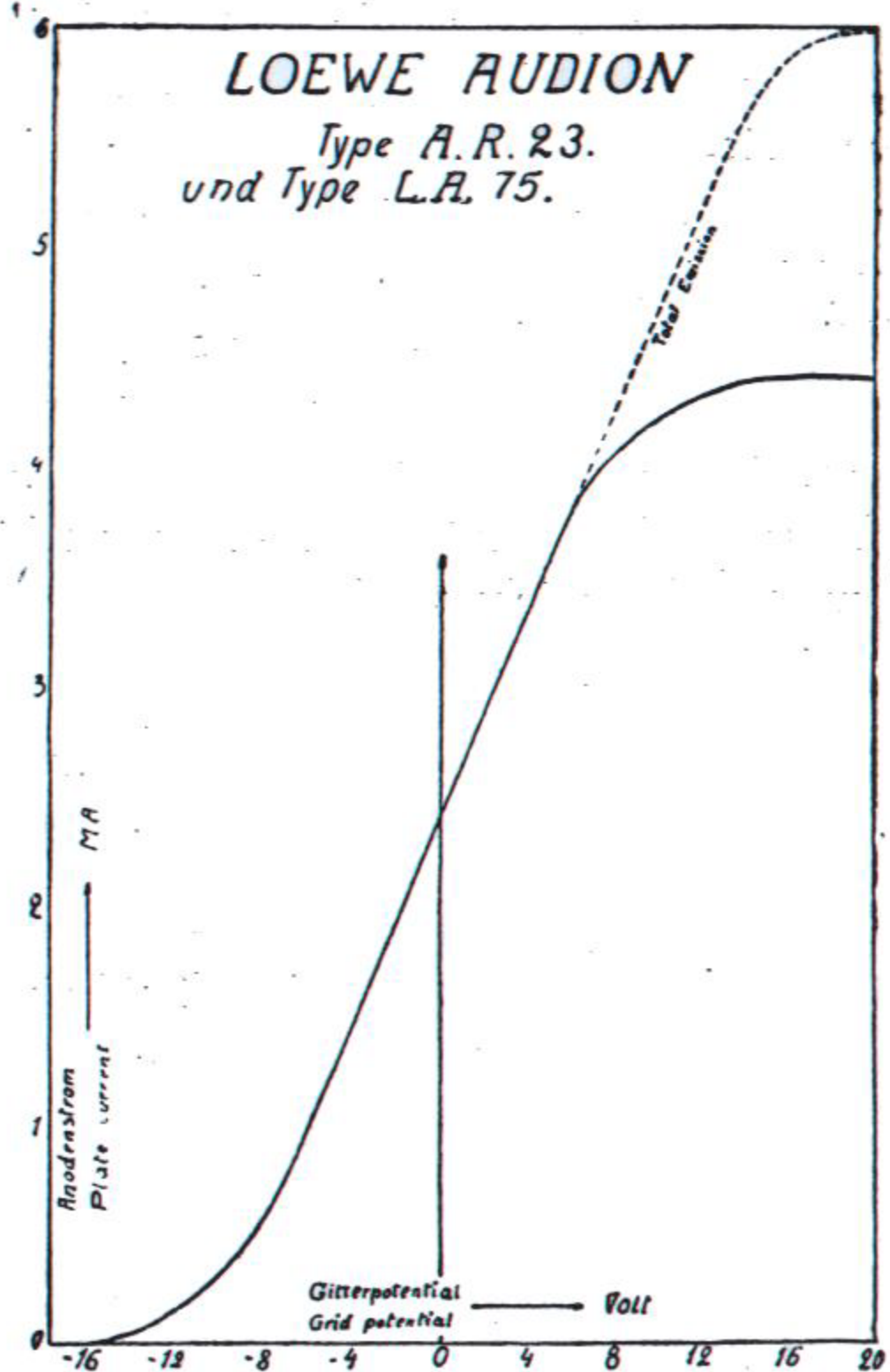
Fig. 48. Charakteristik der Audion-Typen AR 23 und LA 75.
